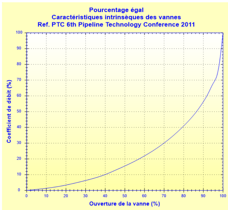
C_{\text{coef Débit}}(O_{\text{uv Vanne}}) ([1] Figure
